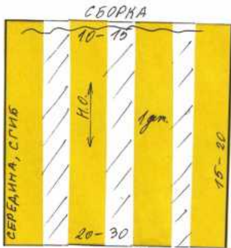
↑ ЗАДНЕЕ ПОЛОТНИЩЕ ЮБКИ
