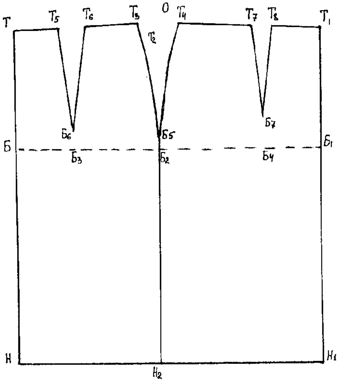
Чертеж в М 1:4 для моделирования
