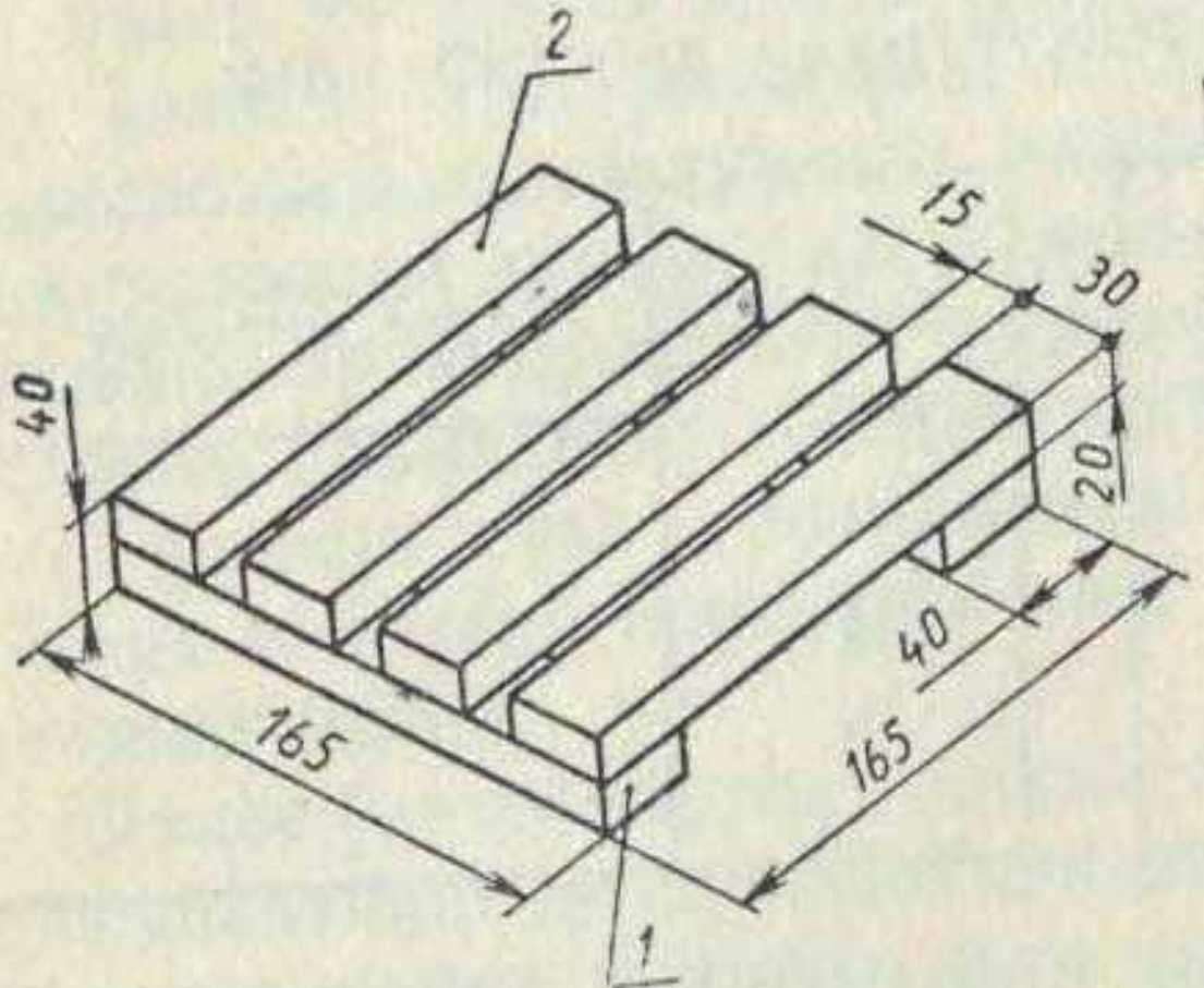
Рис. 1. Подставка для комнатных растений: 1 — ножка; 2 — рейка
