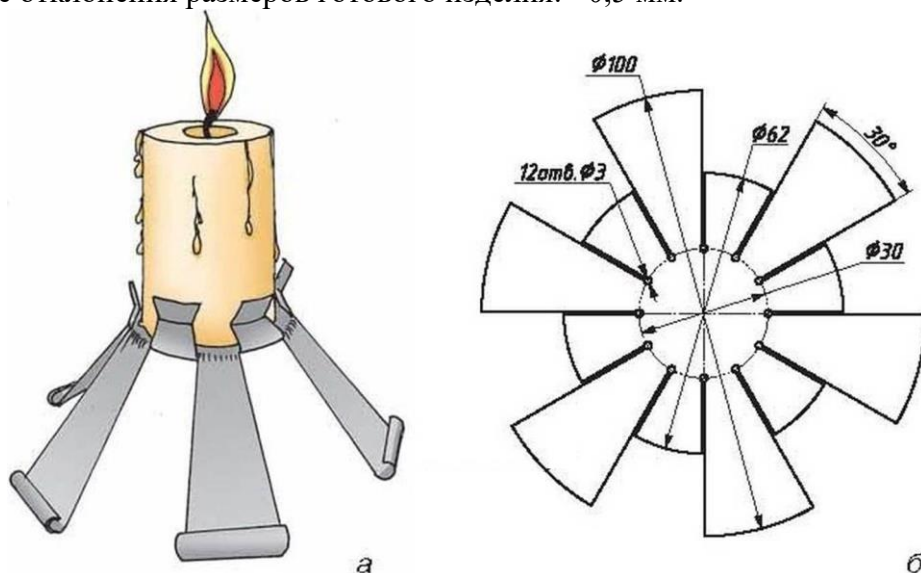
Рисунок 1. Образец подсвечника из тонколистового металла
