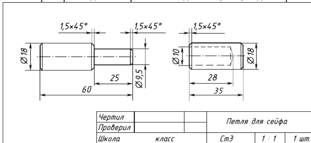
Рис. 1 Петля для сейфа
