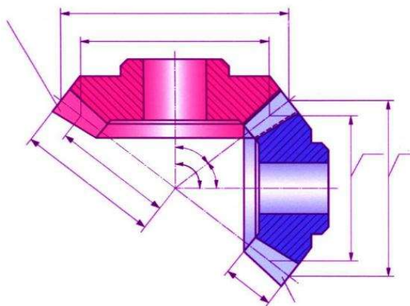
Рис. Коническая зубчатая передача
