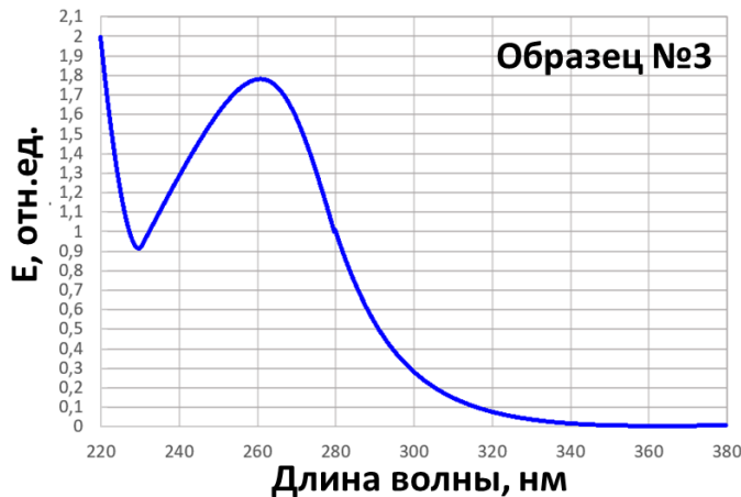
Рисунок 1. Спектры поглощения образцов ДНК. По оси абсцисс – длина волны света, нм (нанометры); по оси ординат – значение поглощения E , отн.ед. (относительные единицы).
