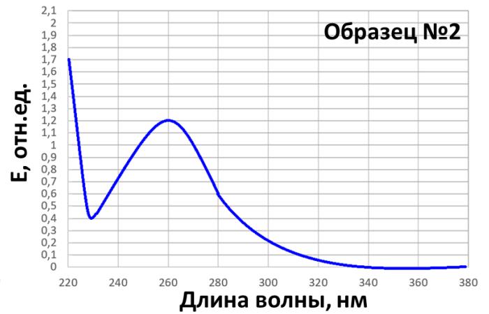
Рисунок 1. Спектры поглощения образцов ДНК. По оси абсцисс – длина волны света, нм (нанометры); по оси ординат – значение поглощения E , отн.ед. (относительные единицы).
