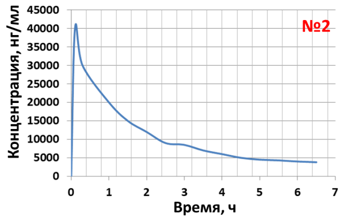
Рисунок 1. Фармакокинетические кривые различных лекарственных препаратов. По оси абсцисс – время, ч (часы), по оси ординат – концентрация препарата в плазме крови: №1 – пг/мл (пикограмм на миллилитр), №2 и 3 – нг/мл (нанogramм на миллилитр).
