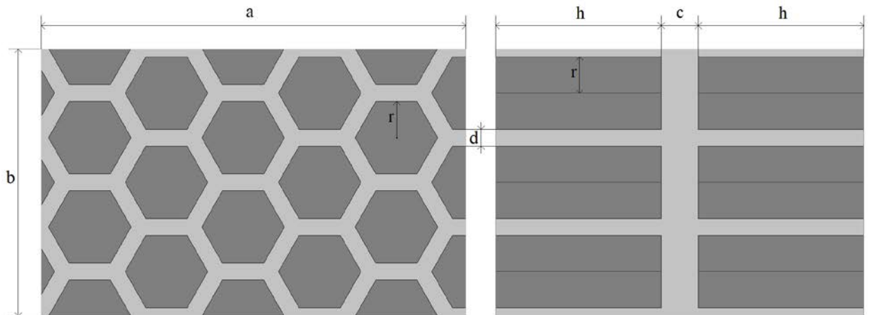
Вид сверху
