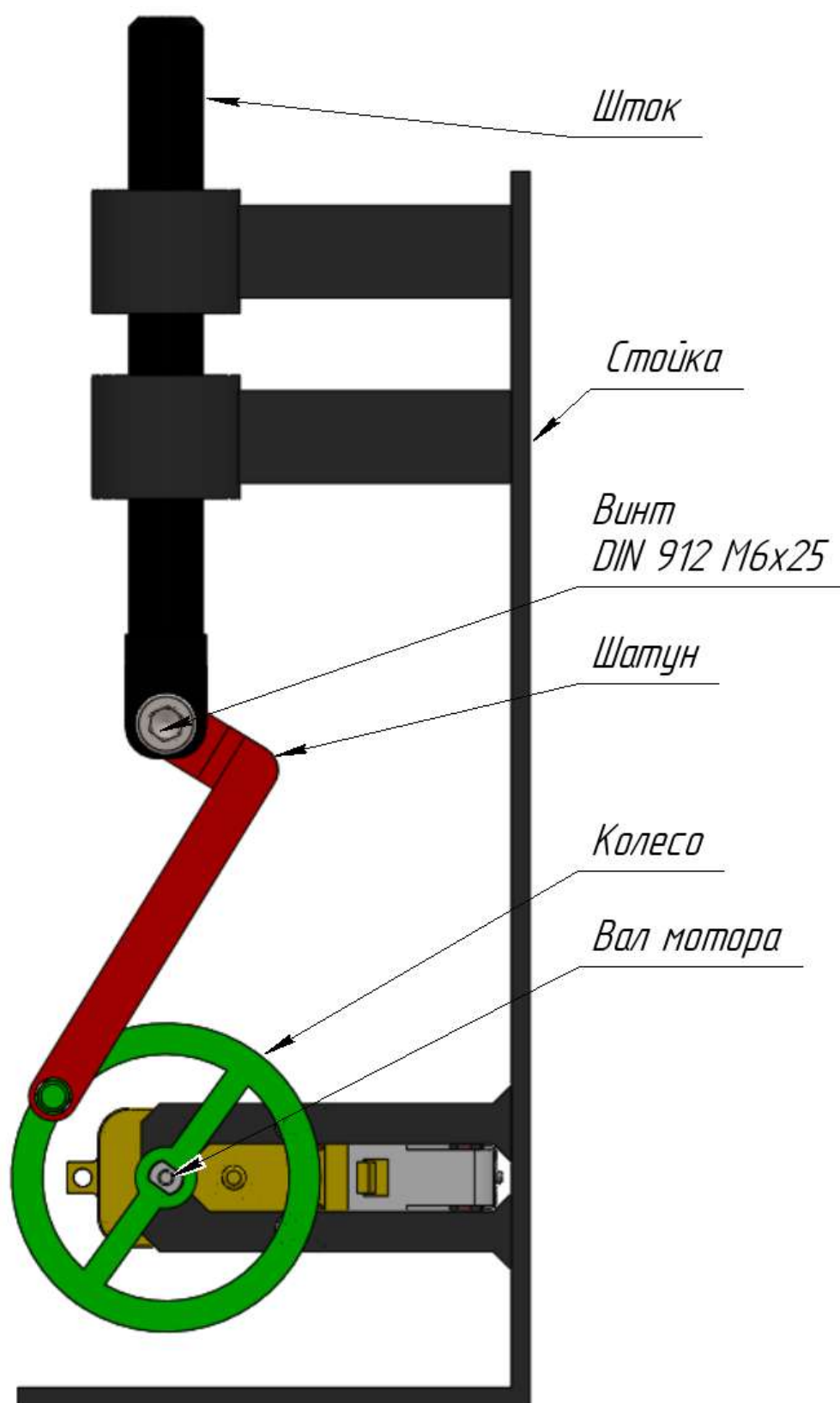
Схема механизма
