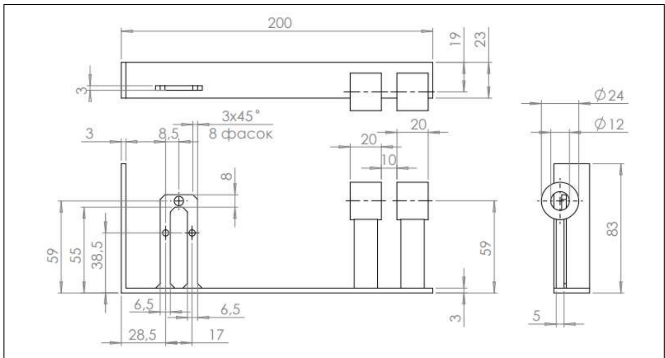
Чертеж стойки
