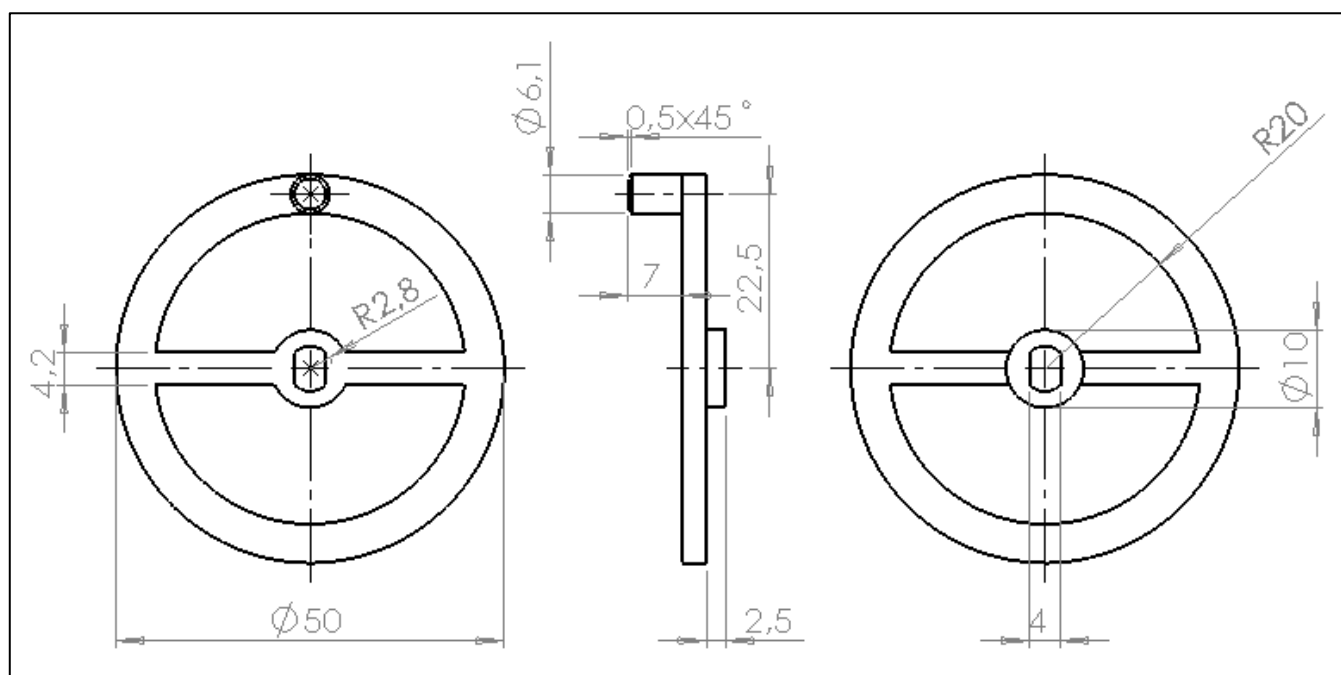
Чертеж колеса
