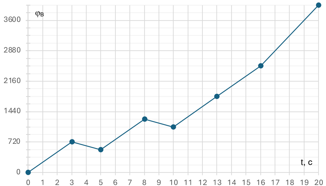
График изменения показаний энкодера мотора В
