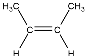
Цис-бутен-2
