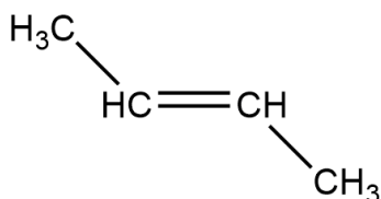
Транс-бутен-2
