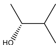
(R)-3-метилбутанол-2
