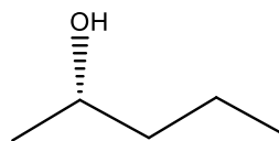
(S)-пентанол-2
