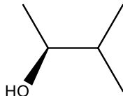
(S)-3-метилбутанол-2
