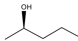
(R)-пентанол-2
