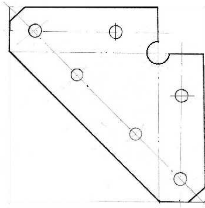
Развертка детали "Скоба угловая"
