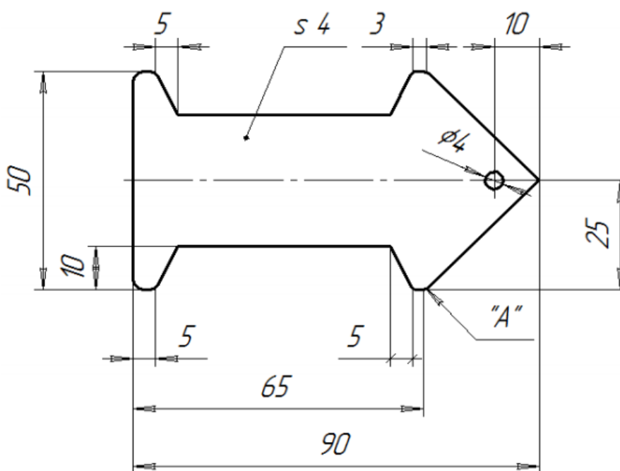
Рис. 1. Чертеж бобины для ниток
