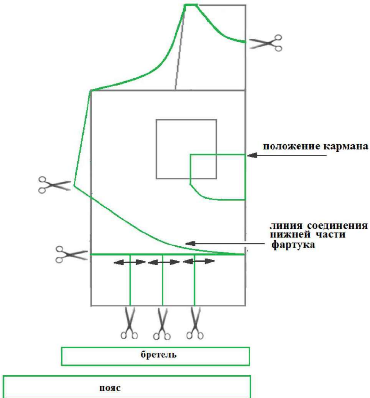
Результат нанесения фасонных линий
