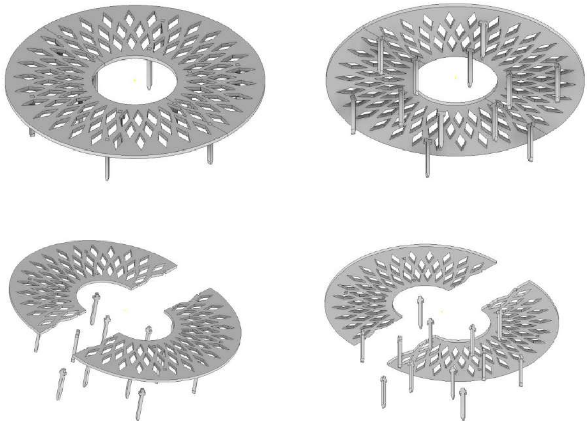
Рисунок 1 – Оригинальная модель защитной сетки для цветочного горшка
