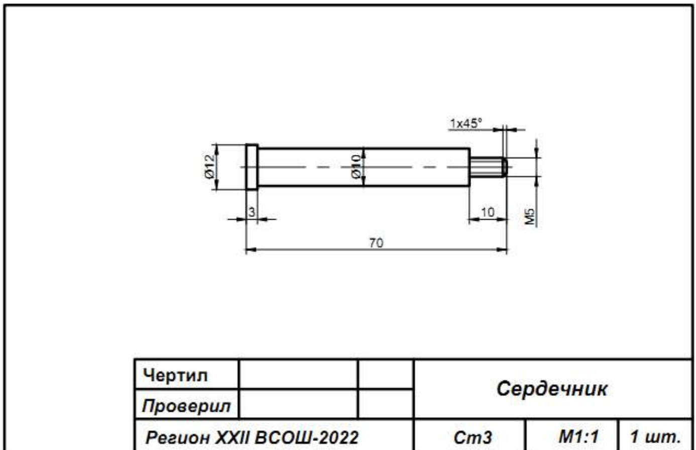
Рис. 1. Чертёж сердечника.
