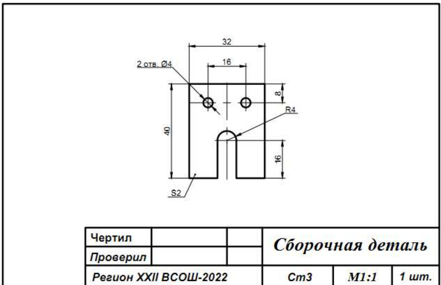
Рис. 1. Чертёж
