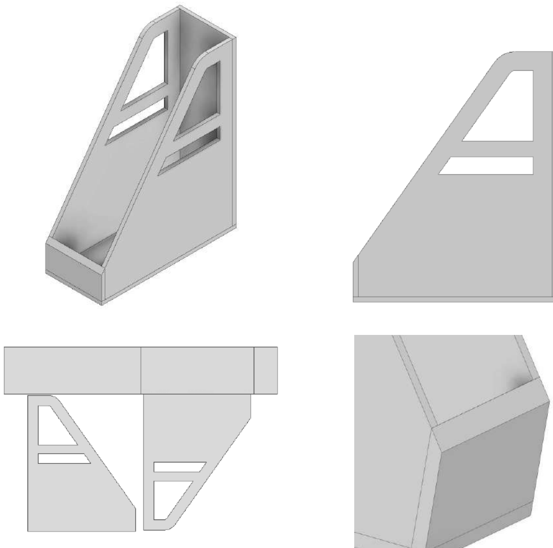
Рисунок 1 – Оригинальная модель изделия
