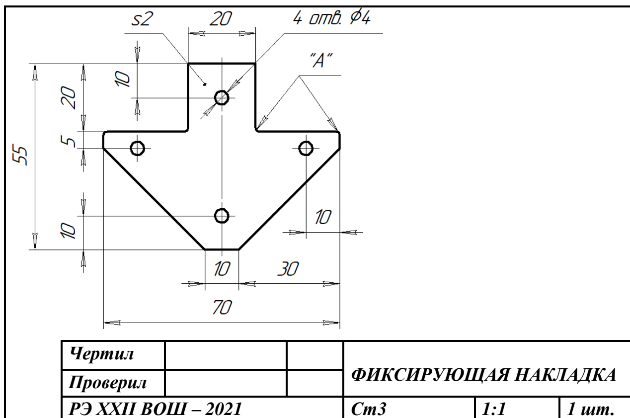
Рис. 1. Чертеж фиксирующей накладки
