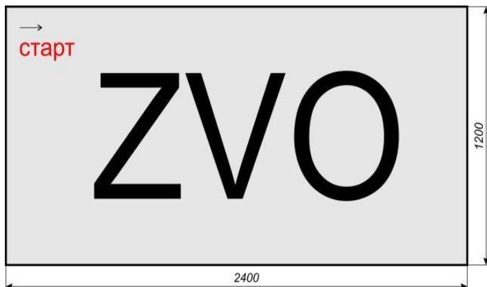
Геометрическая фигура
