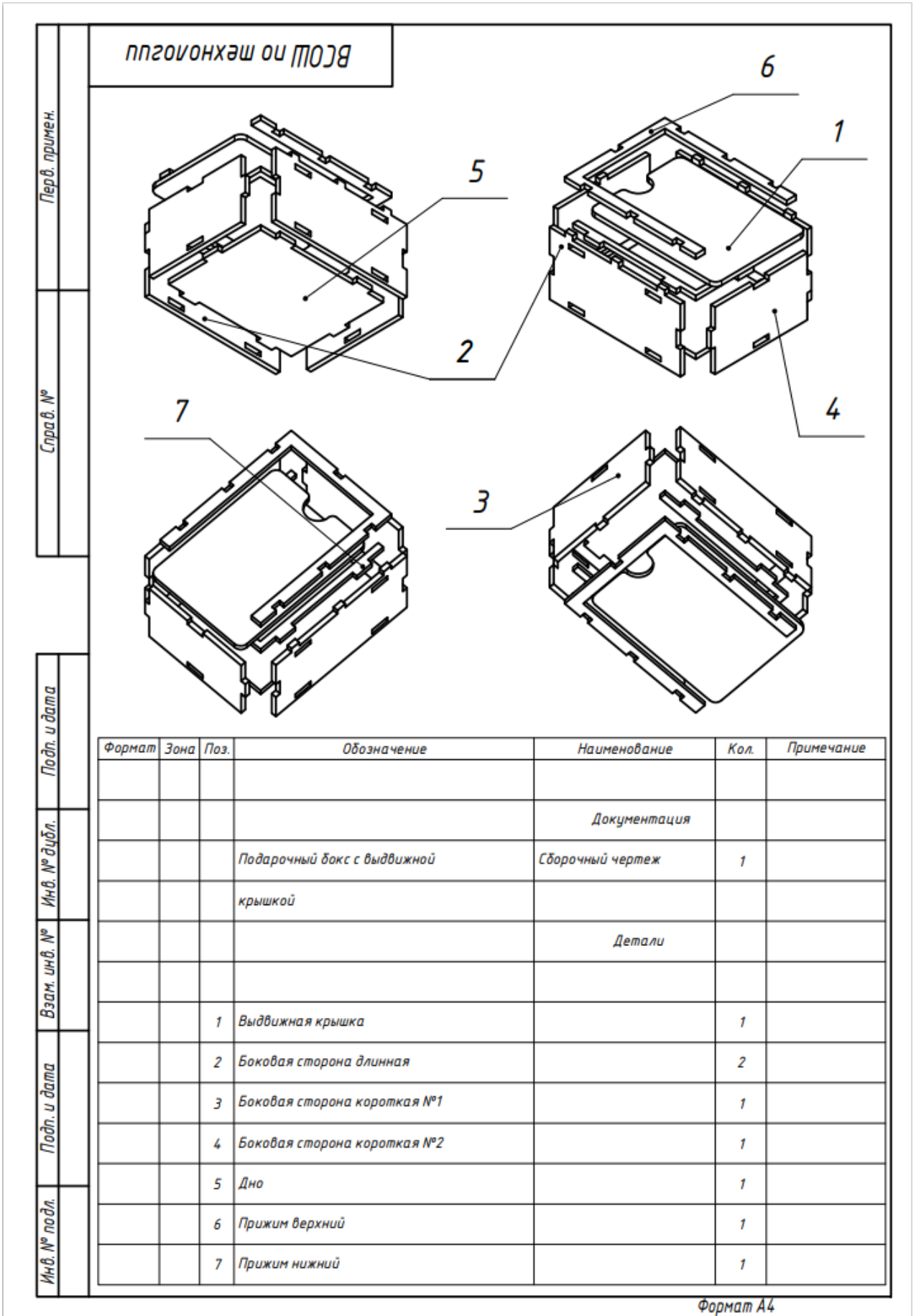
Рисунок 2 – Чертеж изделия
