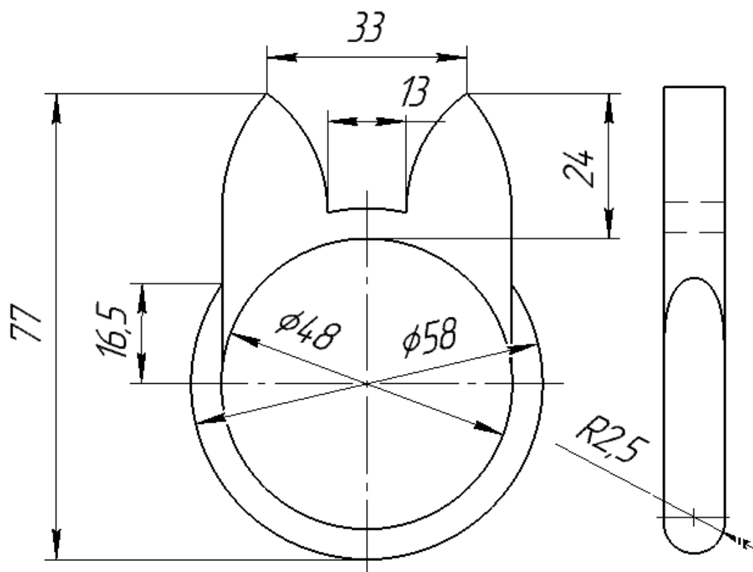
Рисунок 1 - Чертеж изделия
