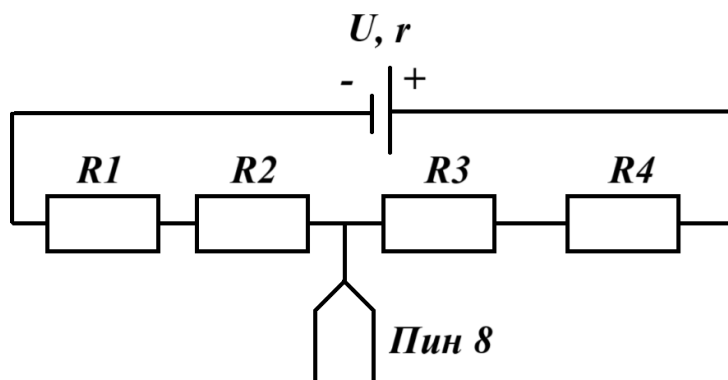
Схема цепи
