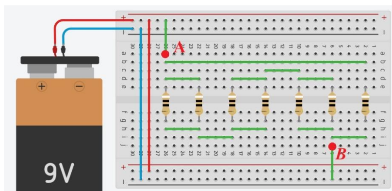
Схема цепи
