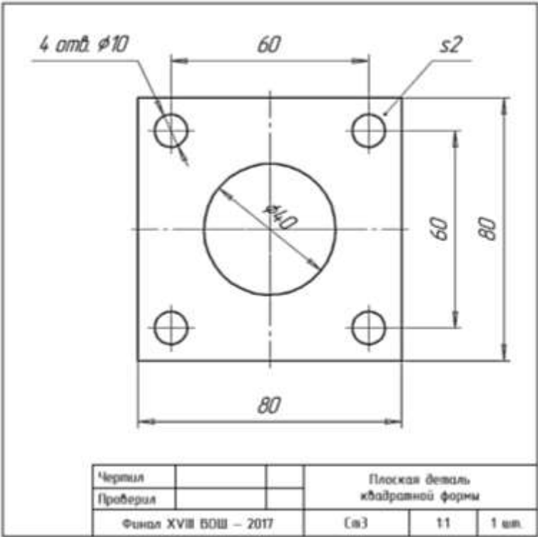
Рис. 1. Образец чертежа плоской детали квадратной формы
