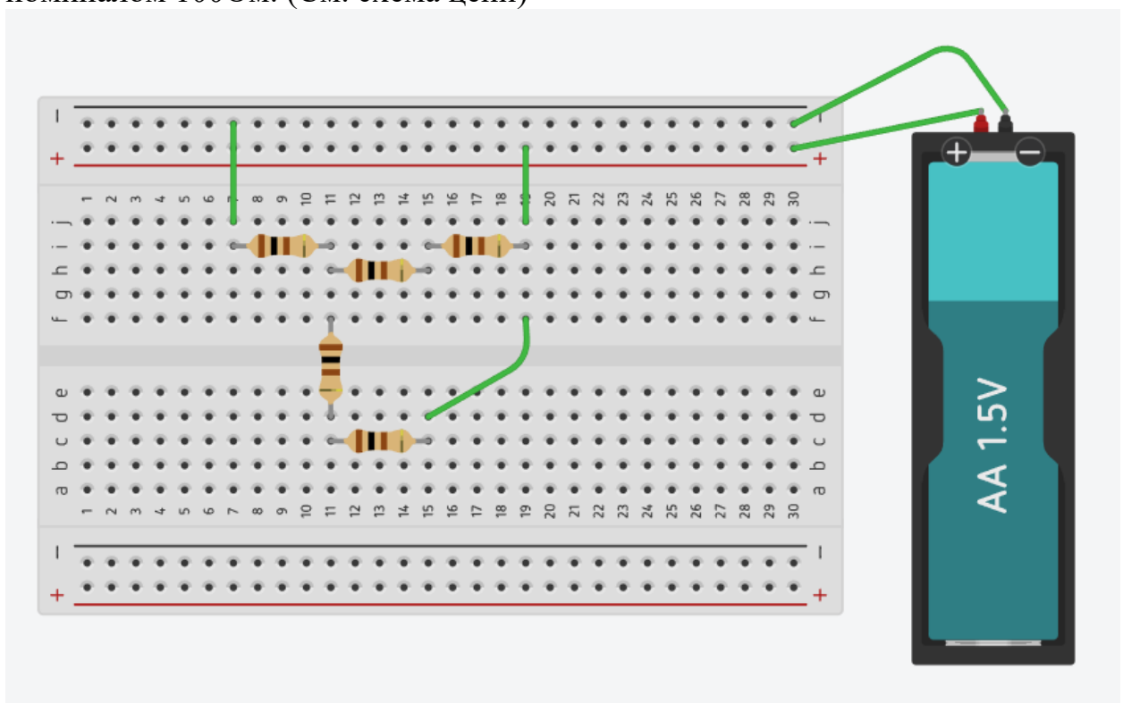
Схема цепи
