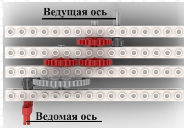
Схема передачи
