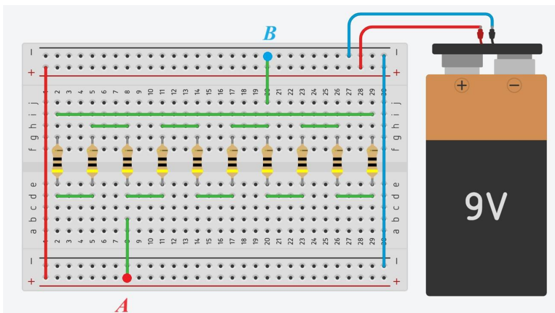
Схема цепи
